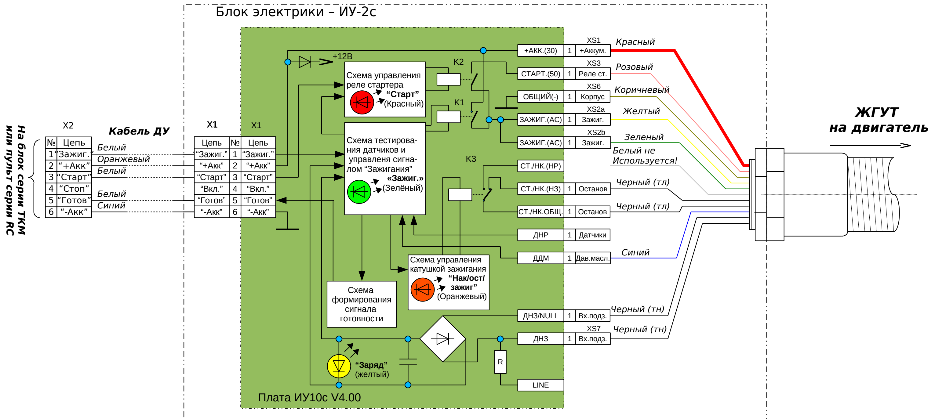
Рис.П1.1. Электрическая схема подключения комплекта ИУ-2с (Часть 1).
